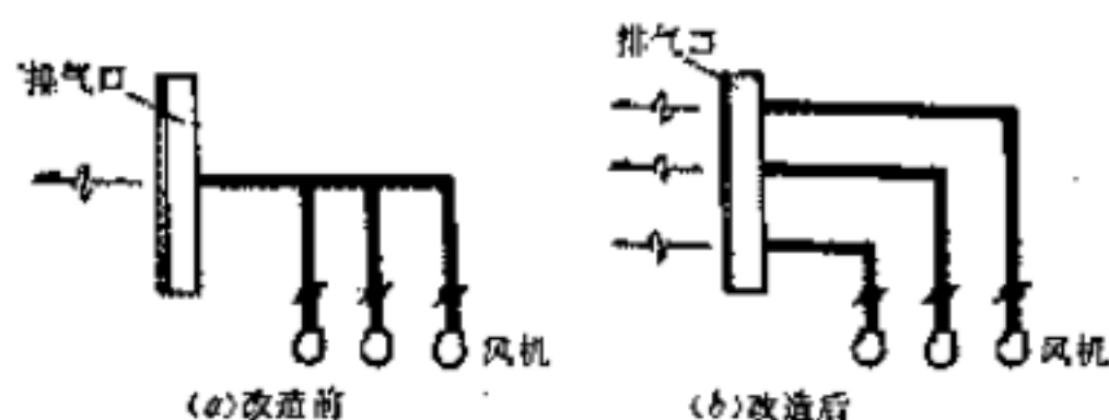
图 2.3.4-2 排气合流相互干扰（二）
