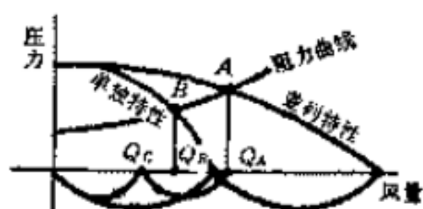
图 2.3.4-3 风机并联运行特性
