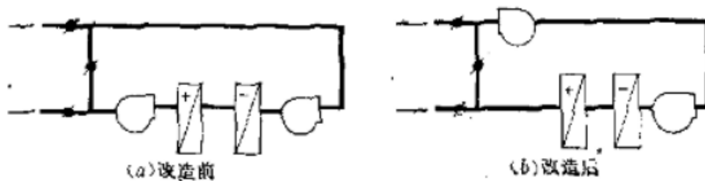
图 2.3.2-1 双风机的布置
