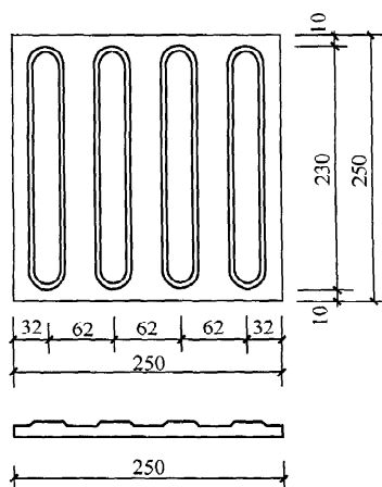
图 3-3 行进盲道
