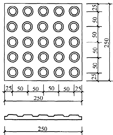
图 3-4 提示盲道
