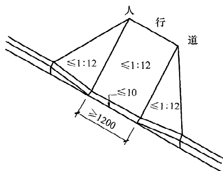
图 3-2 三面坡缘石坡道
