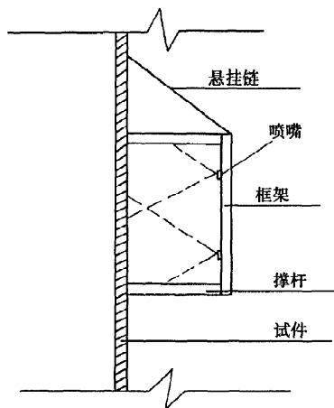
图 C.0.2 幕墙淋水试验装置安装示意
