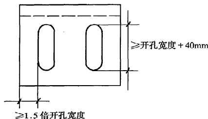
图 2.6.3 转接件、连接件的开孔示意
