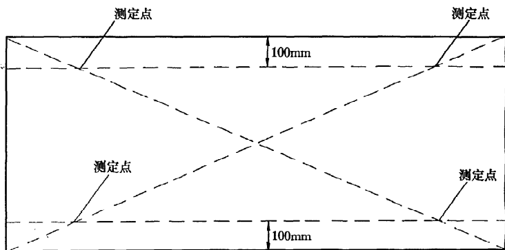
图 B.0.1-1 表面应力测量点示意
