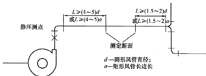
图 3.2.3 测定断面位置选择示意
