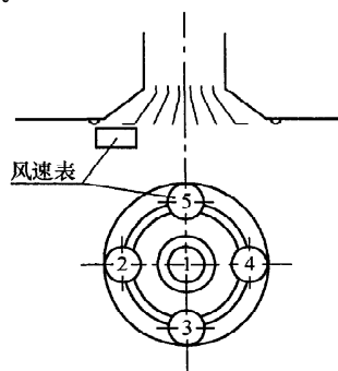
图 3.4.3-2 用风速仪测定散流器出口平均风速
