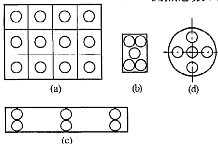
图 3.4.3-1 各种形式风口测点布置
