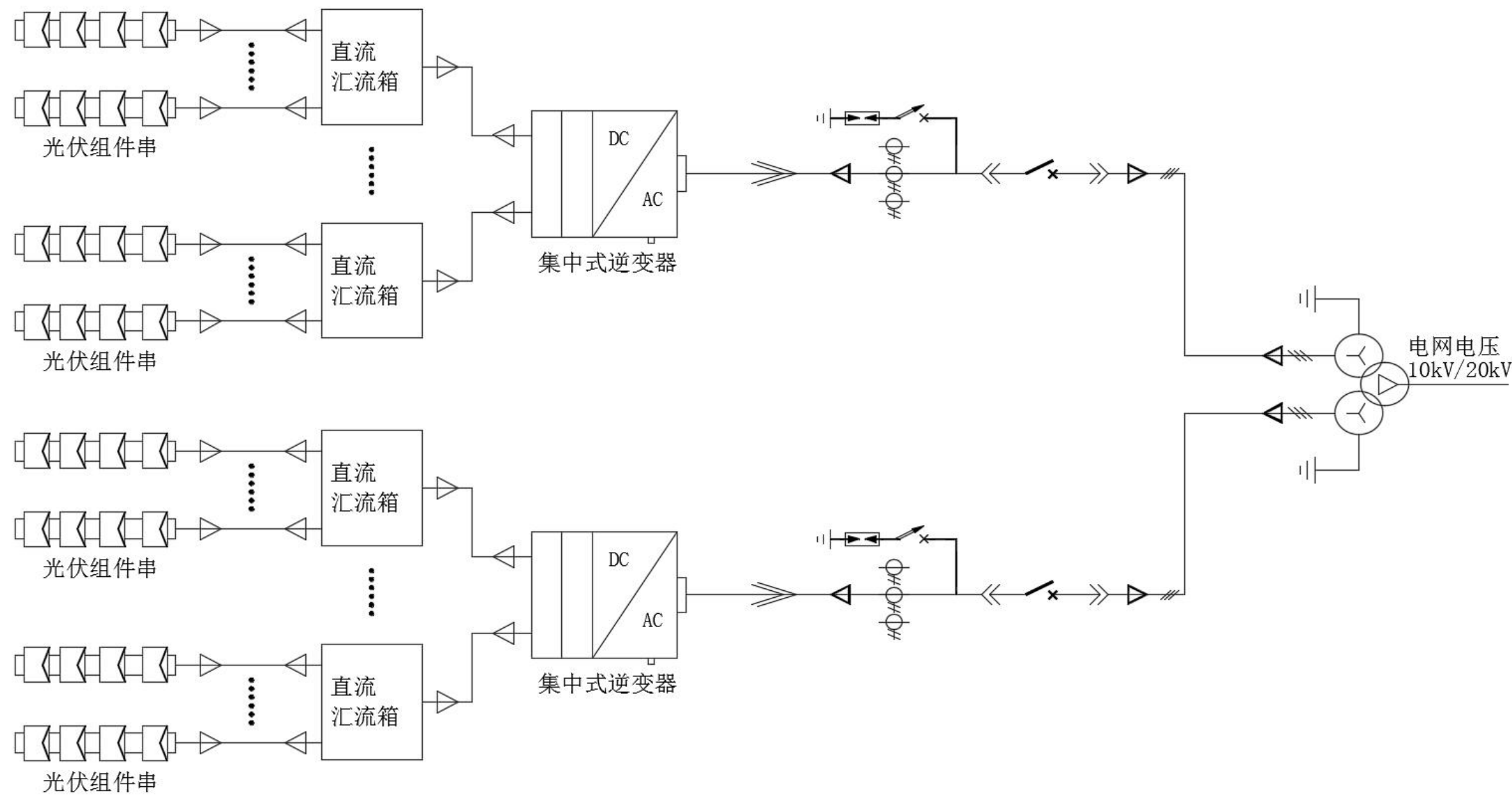
10（20）kV并网方案（一）
