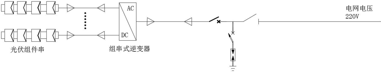
220V并网方案（二）
