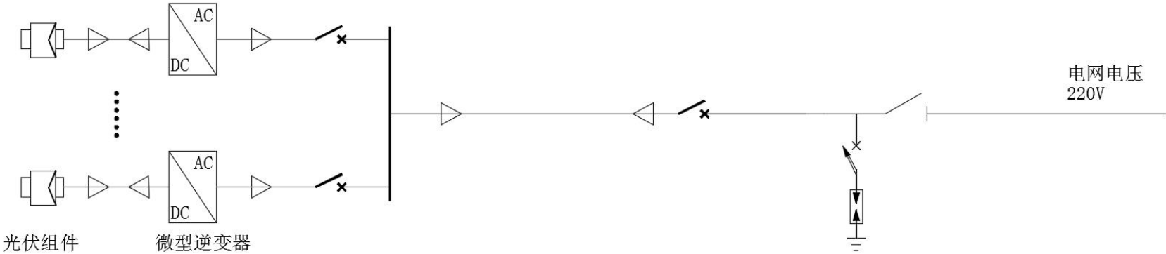
220V并网方案（一）
