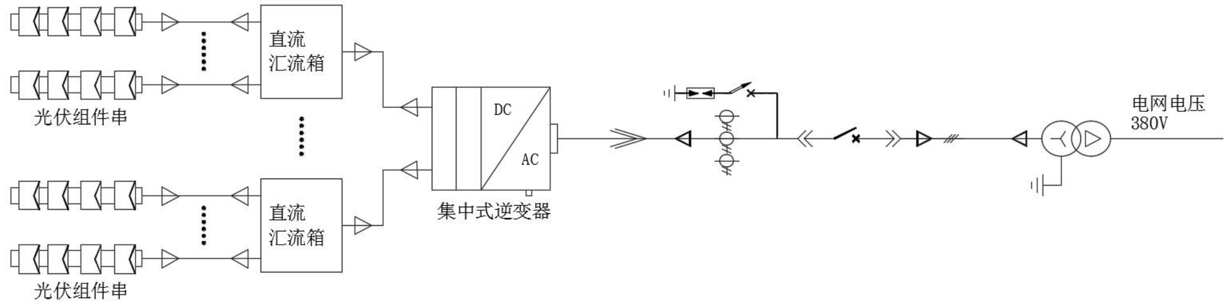
380V并网方案（一）
