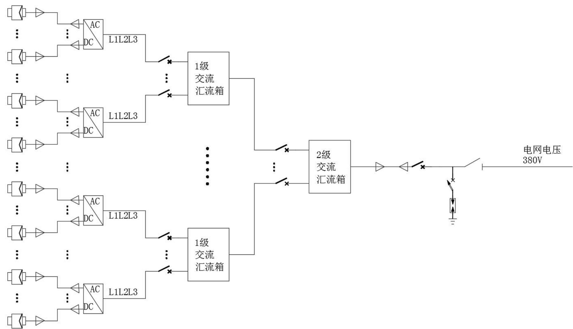
380V并网方案（三）
