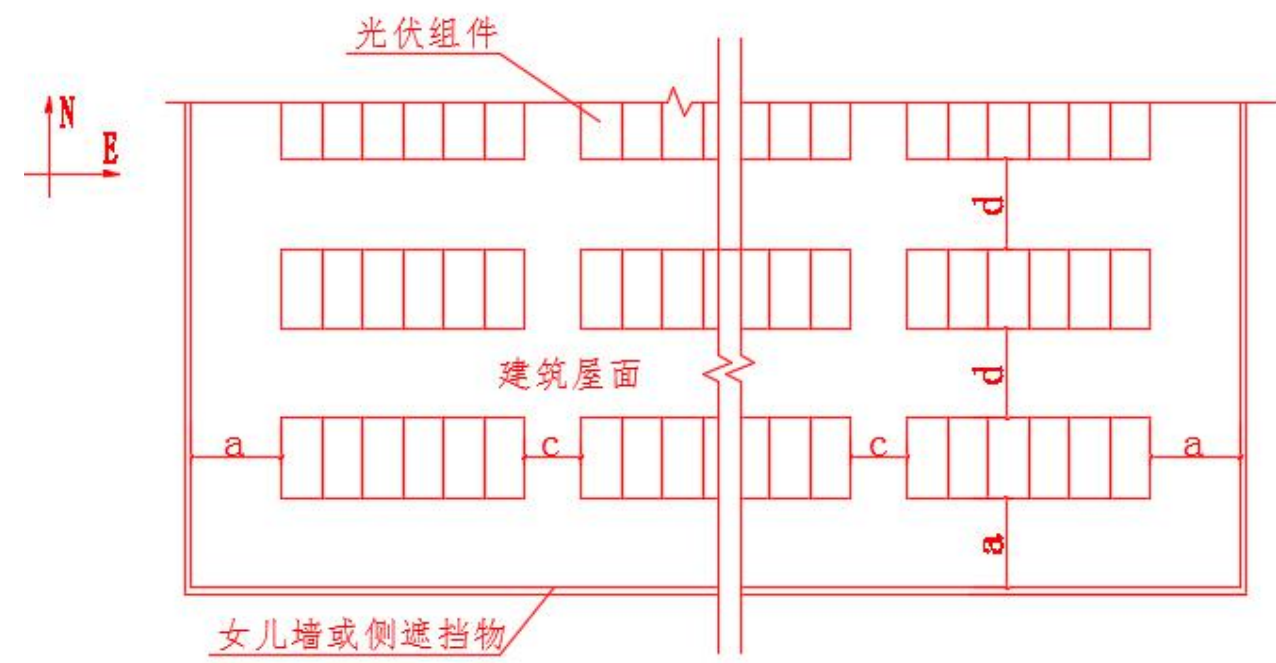
屋面光伏组件阵列排布平面图
