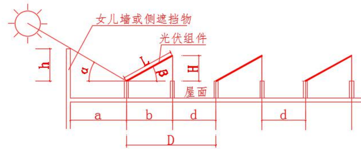
屋面光伏组件阵列排布剖面图
