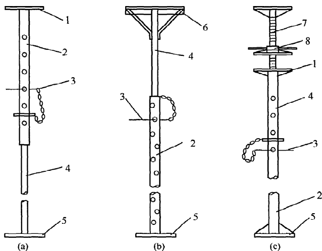
图 5.2.5-1 钢管立柱类型 (一)
