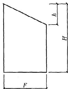
图 4.1.1 混凝土侧压力 计算分布图形
