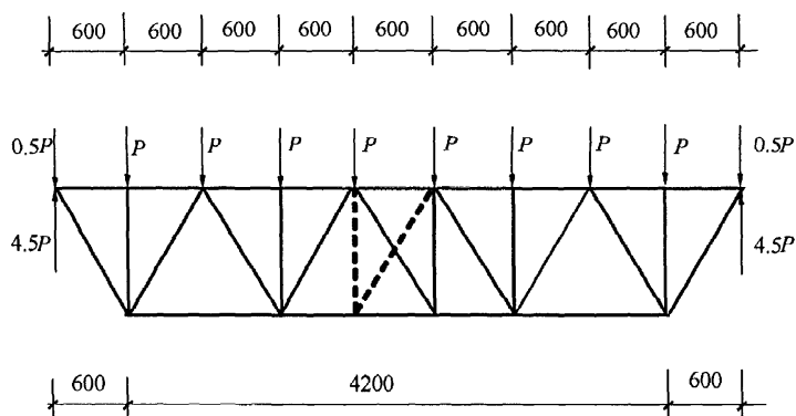
图 5.2.2-3 可调桁架跨长计算简图示意
