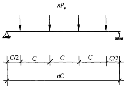
图 5.2.2-5 桁架节点集中荷载布置图 (中间等分)
