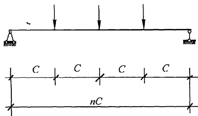
图 5.2.2-4 桁架节点集中荷载布置图 (全跨等分)
