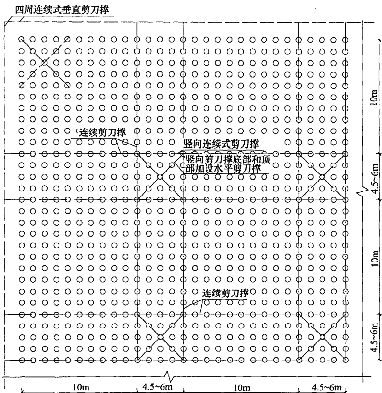
图 6.2.4-3 剪刀撑布置图 (三)
