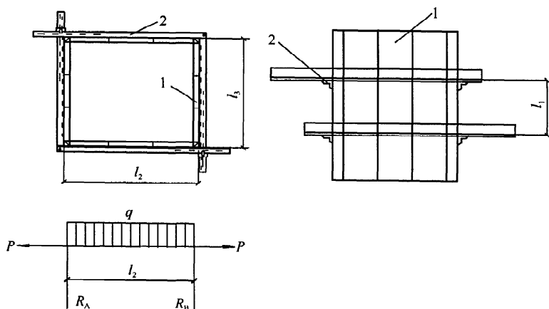
图 5.2.4 柱箍计算简图
