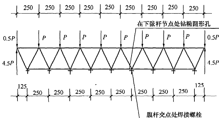
图 5.2.2-2 曲面可变桁架计算简图示意
