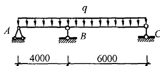
图 C.2-1 二跨不等跨连续梁计算简图
