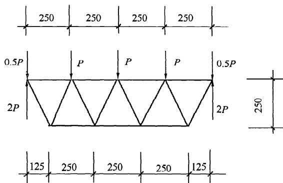
图 5.2.2-1 轻型桁架计算简图示意
