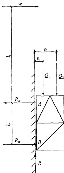
图 5.3.5-1 附墙架与墙 连接螺栓计算简图
