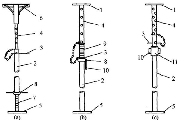
图 5.2.5-2 钢管立柱类型 (二)
