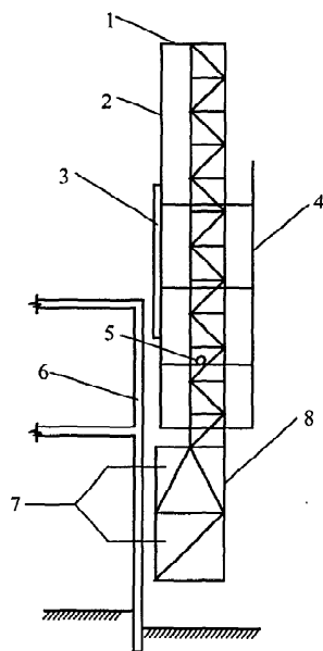
图 5.3.1 爬模组成
