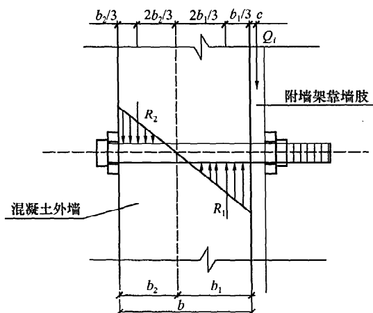
图 5.3.5-2 螺栓孔混凝土承压计算
