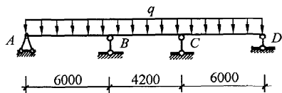
图 C. 2-2 三跨不等跨连续梁计算简图
