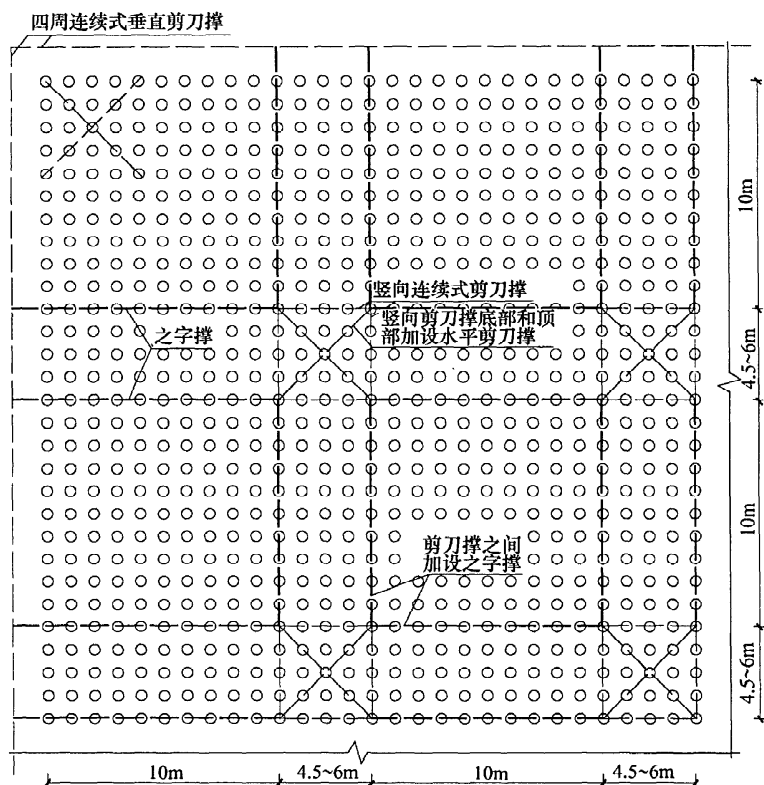
图 6.2.4-2 剪刀撑布置图 (二)
