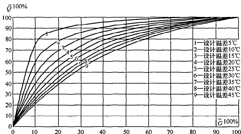
图 2 散热器流量和散热量的关系曲线
