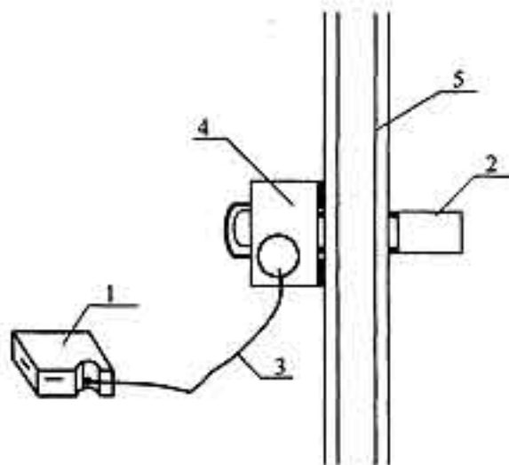
图 B.0.4 玻璃透射比现场检测示意图
