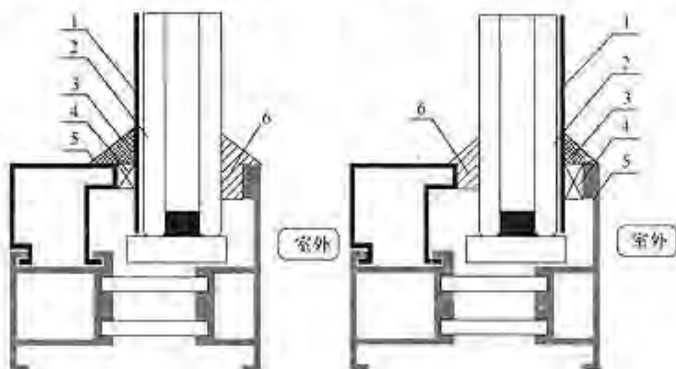
图 4.2.3-1 安全贴膜与门窗结构体系的连接
