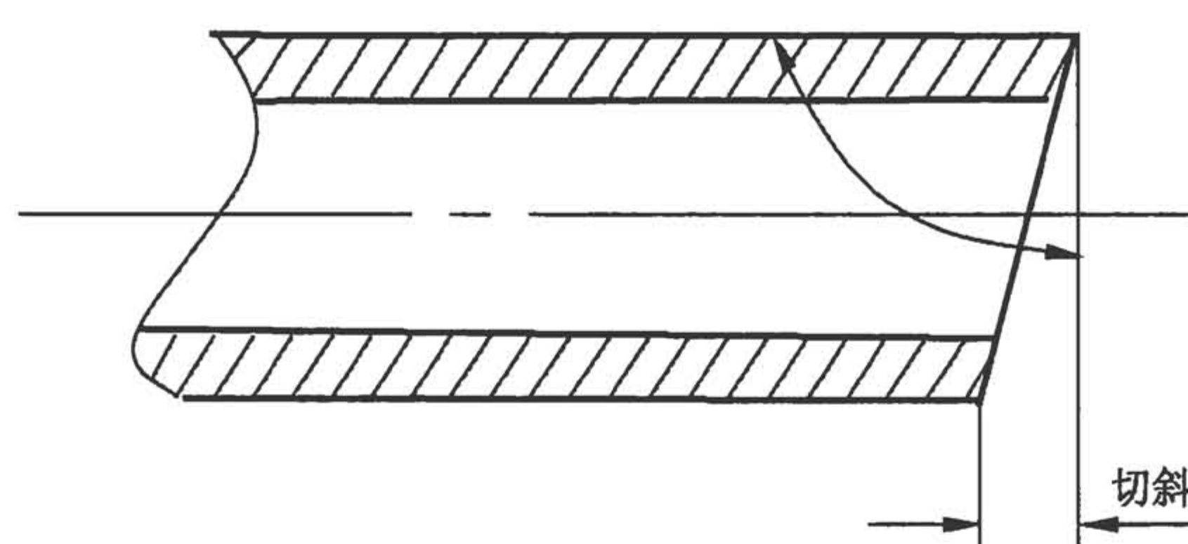
图 1 切斜示意图
