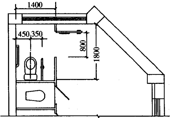
图 7.8.1-3 新建无障碍厕位
