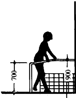
卫生间墙间扶手
