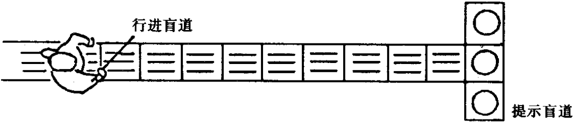
图 4.2.3-1 盲道起点与终点提示盲道
