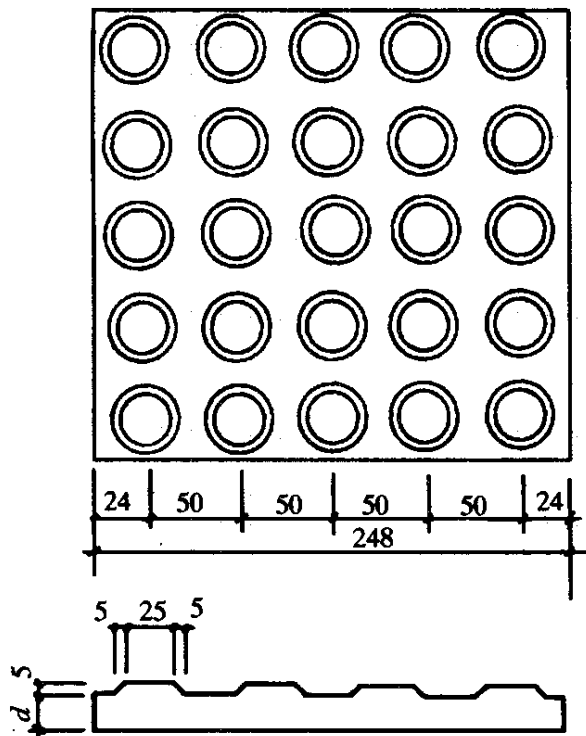
图 4.2.3-4b 人行横道入口提示盲道
