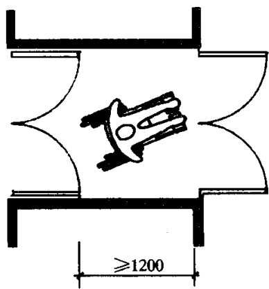
图 7.1.5-1 小型公建门厅门扇间距
