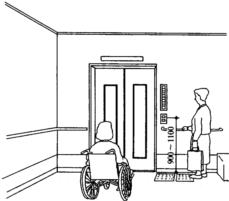
图 7.7.2 候梯厅
