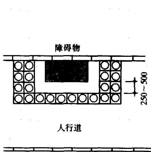
图 4.2.3-3 人行道障碍物的提示盲道
