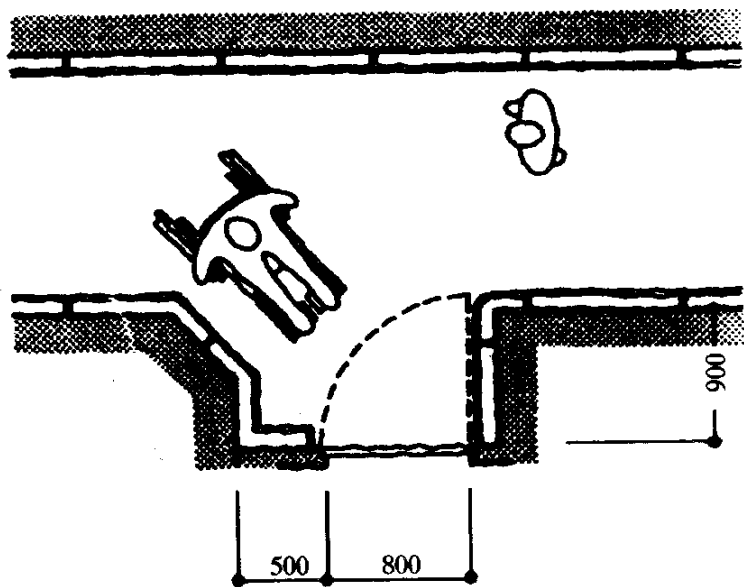
图 7.3.5 走道的凹室
