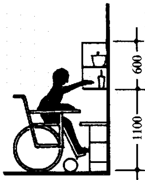
吊柜高度位置
