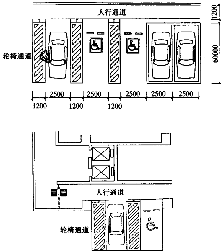
图 7.11.3 停车车位及轮椅通道
