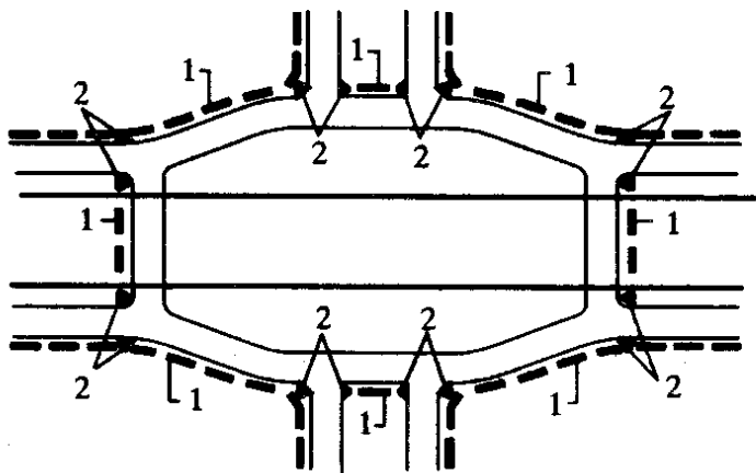
图 4.5.2-2 立体交叉中非机动车道的无障碍设施
