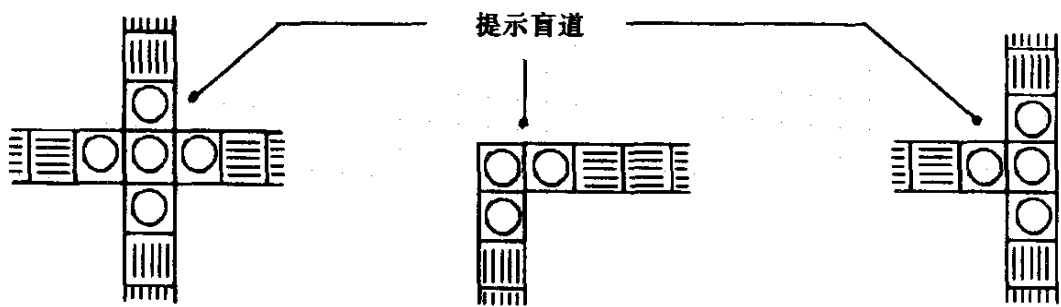
图 4.2.3-2 盲道交叉提示盲道
