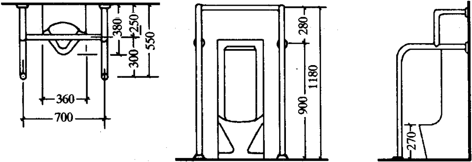
图 7.8.1-1 落地式小便器安全抓杆
