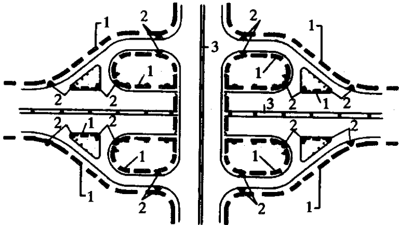
图 4.5.2-1 立体交叉无障碍设施布置 1—盲道；2—缘石坡道；3—隔离带
