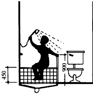
淋浴池侧做坐台及扶手
