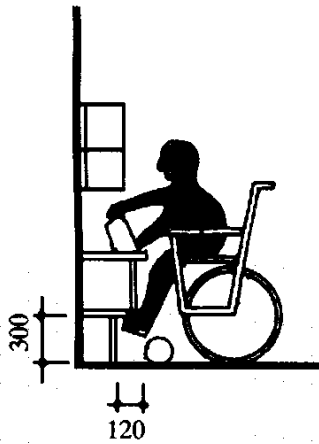
切菜台下面去掉 300
