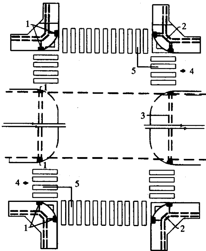
图 4.5.2-3 菱形立交中无障碍设施布置
