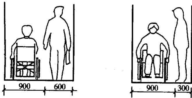
图 11 走道宽度
