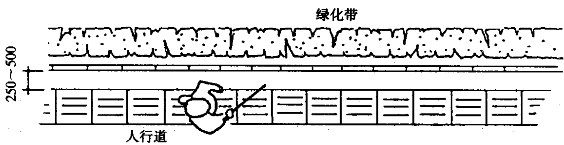
图 4.2.2-1 缘花台的行进盲道
