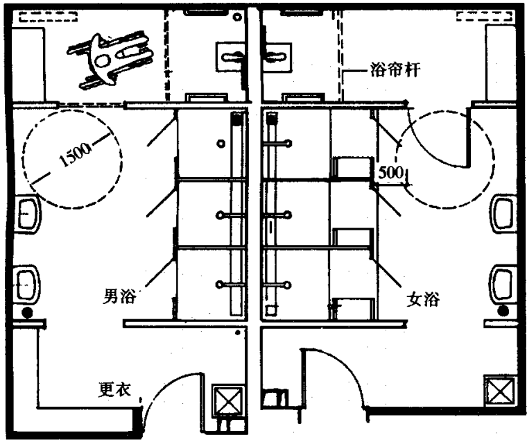
图 17 残疾人使用的淋浴间 (mm)
