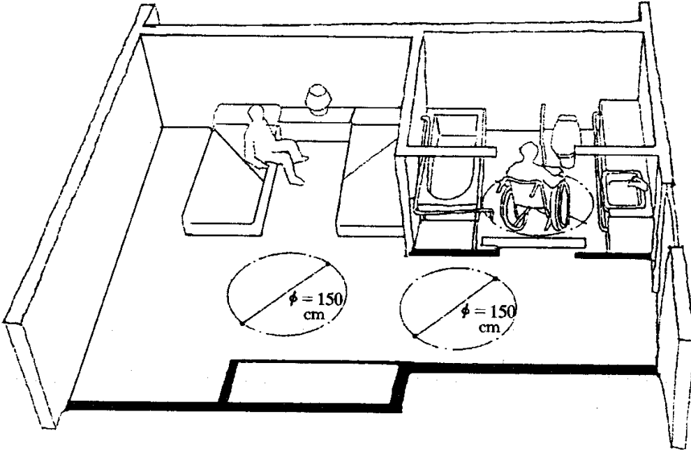
图 19 残疾人客房
