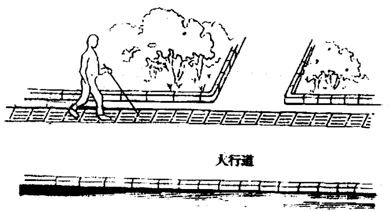
图 4 人行道外侧沿花台的盲道
