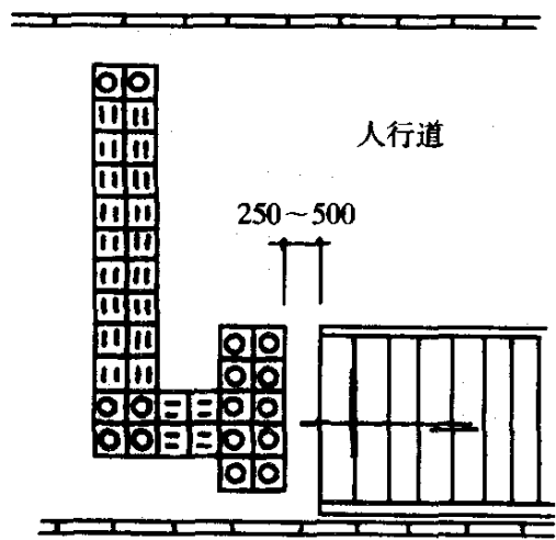
图 4.2.3-4a 地下铁道入口提示盲道
