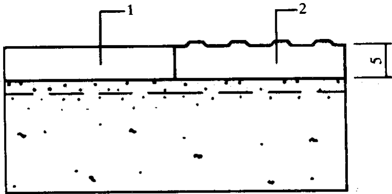
图 4.2.1-3 人行道砖与盲道砖的连接
