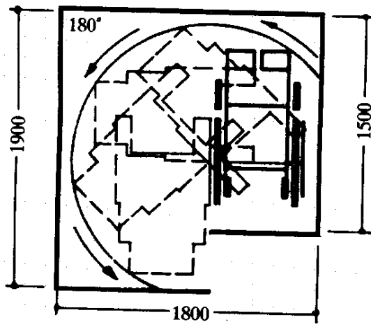
e 以一个轮为中心旋转 180°所需最小面积为 1800mm × 1900mm
