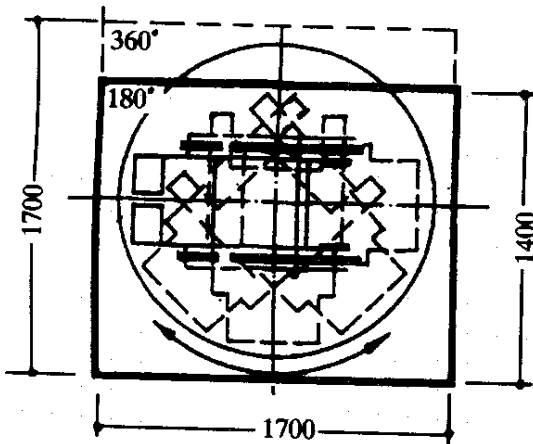
c 以两轮中央为中心,旋转 180°所需最小面积为 1400mm × 1700mm
