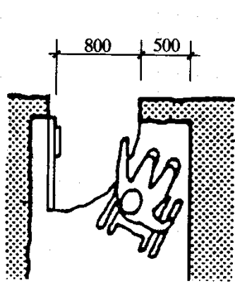
图 7.4.1-1 门把手一侧 墙面宽度 (mm)
