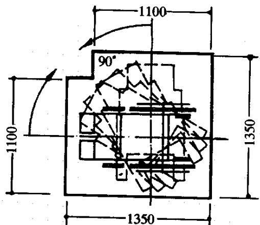
b 轮椅旋转 90°所需最小面积为 1350mm × 1350mm
