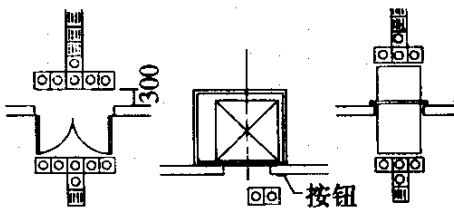
c. 门前及电梯盲道
