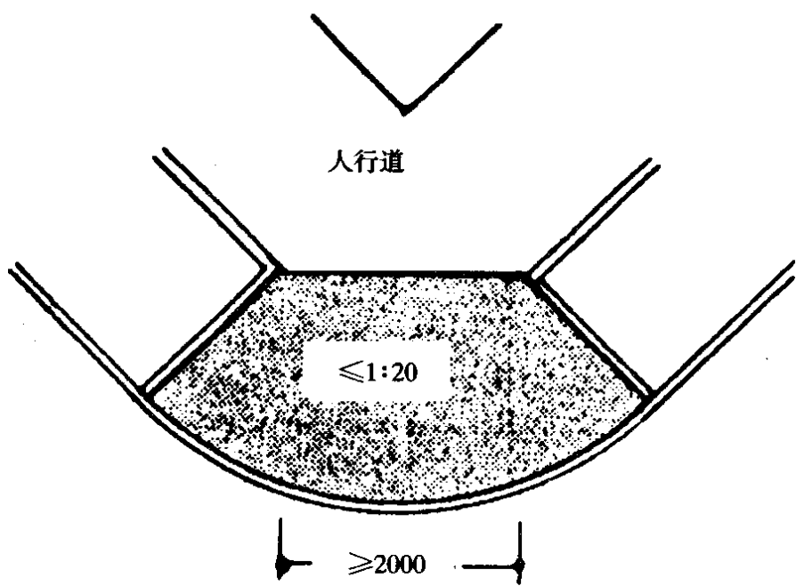
图 4.1.2-5 转角处单面直线缘石坡道
