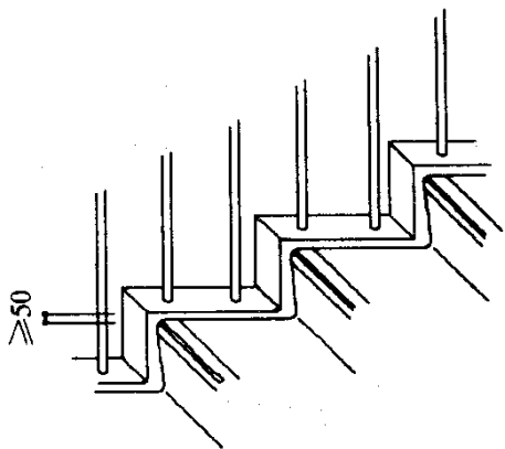
图 7.5.1-4 踏步安全挡台
