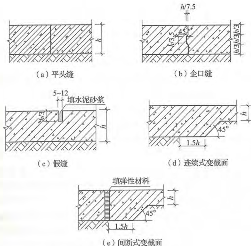
图 6.0.3 混凝土垫层缩缝
