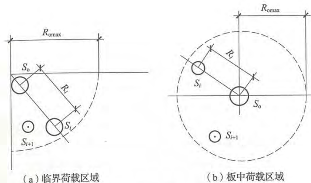
图 C. 2. 9 荷载区域
